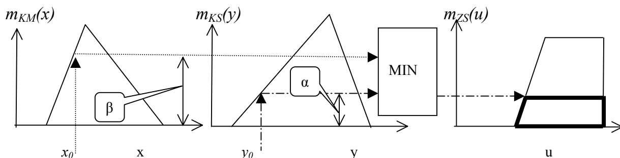
Obr.6. Nalezení výstupní množiny pro jedno pravidlo a dvourozměrnou závislost
