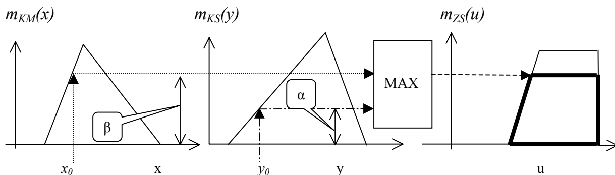
Obr.7. Nalezení výstupní množiny pro jedno pravidlo a dvourozměrnou závislost s operátorem OR
