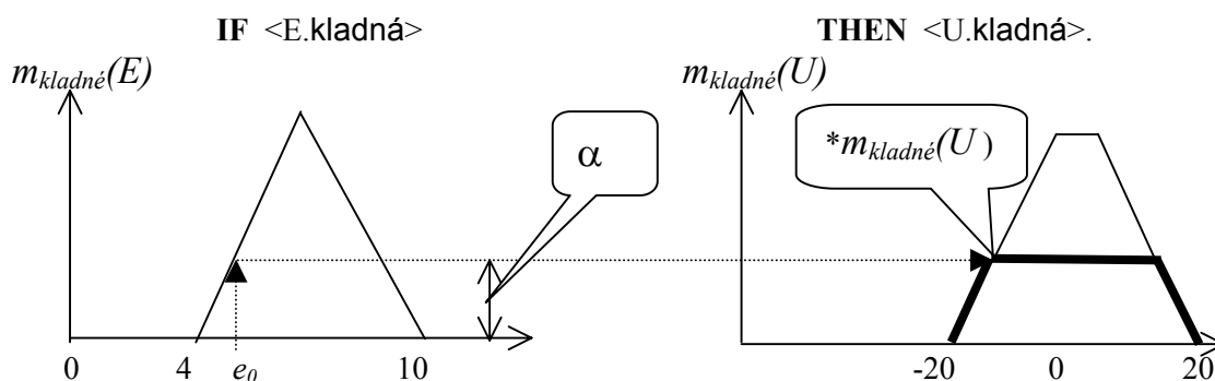
Obr.5 Mamdaniho implikace na jednorozměrné závislosti
