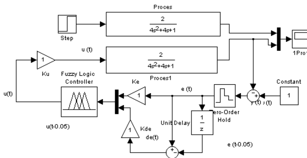
Obr.18 Základní struktura zpětnovazebního obvodu s fuzzy regulátorem
