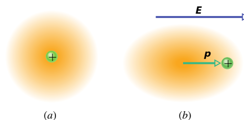
Obr. 25.12 (a) Atom s kladně nabitým jádrem (zeleně) a záporně nabitými elektrony (zlatě stínované). Střed kladného náboje jádra splývá se středem záporně nabitých elektronových obalů atomu. (b) Je-li atom umístěn do vnějšího elektrického pole, jsou elektronové orbity deformovány a tím se středy kladného a záporného náboje oddálí. Atom tak získá elektrický dipólový moment. Deformace elektronových drah je značně přehněná.
