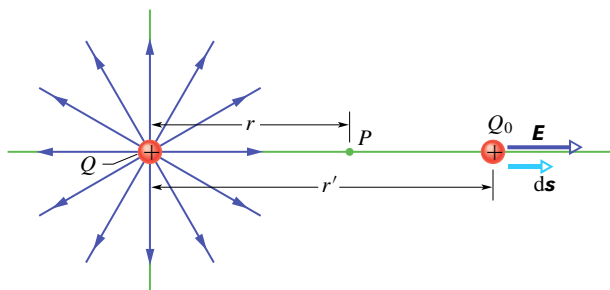
Obr. 25.7 Kladný bodový náboj Q vyvolává v bodě P elektrické pole o intenzitě \mathbf{E} a potenciálu \varphi . Potenciál v bodě P určujeme s pomocí testovací částice s nábojem Q_0 , kterou přemísťujeme z bodu P do nekonečna. Je znázorněno infinitesimální posunutí částice o d\mathbf{s} ve vzdálenosti r' od bodového náboje.
