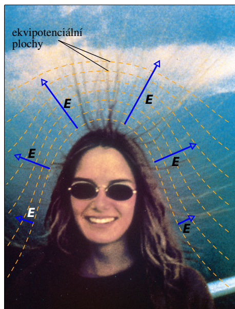
Obr. 25.4 Schémata doplněná fotografie z úvodní strany této kapitoly ukazuje důsledek působení nabitého mraku, který vytvořil silné elektrické pole o intenzitě E blízko hlavy ženy. Mnohé prameny jejích vlasů se natáhly podél směru elektrického pole, které je vždy kolmé k ekvipotenciálním plochám a silnější je tam, kde jsou tyto ekvipotenciální plochy těsněji u sebe, tj. v tomto případě nad temenem hlavy ženy.
