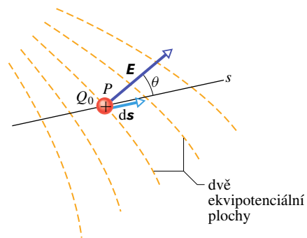
Obr. 25.15 Testovací náboj Q_0 se posune o d\mathbf{s} od jedné ekvipotenciální plochy ke druhé. Vektor posunutí d\mathbf{s} svírá úhel \theta se směrem vektoru intenzity elektrického pole \mathbf{E} .
