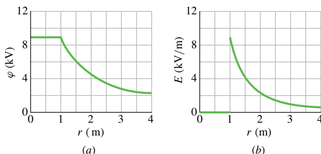
Obr. 25.19 (a) Průběh potenciálu \varphi(r) nabité kulové plochy. (b) Průběh velikosti intenzity elektrického pole E(r) stejné kulové plochy. Na povrchu koule je intenzita nespojité.
