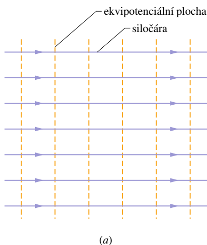
Obr. 25.3 Elektrické siločáry (fialově) a příčné řezy ekvipotenciálních ploch (zlatě) (a) v homogenním elektrickém poli, (b) v elektrickém poli bodového náboje, (c) v poli elektrického dipólu.
