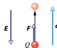
Obr. 25.1 Příklad 25.1. Elektron v atmosféře se přemísťuje svisle vzhůru do vzdálenosti d vlivem elektrostatické síly \mathbf{F} = Q\mathbf{E} .
