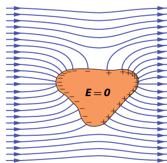
Obr. 25.21 Nenabitý vodič je vsunut do vnějšího elektrického pole. Volné elektrony vodiče se rozdělí po jeho povrchu tak, jak je naznačeno, a zcela zruší elektrické pole uvnitř vodiče. Siločáry výsledného pole těsně nad povrchem vodiče jsou kolmé k jeho povrchu.
