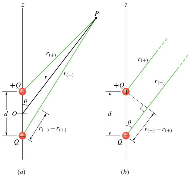
Obr. 25.11 (a) Bod P je ve vzdálenosti r od středu O elektrického dipólu. Úsečka OP svírá s osou dipólu úhel \theta . (b) Je-li bod P velmi daleko od dipólu, jsou úsečky r_{(+)} a r_{(-)} přibližně rovnoběžné s úsečkou OP a čárkovaná černá úsečka je přibližně kolmá k úsečce r_{(-)} .
