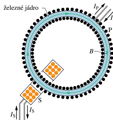
Obr. 32.11 Rowlandův prstenec; užívá se k měření B ve feromagnetických materiálech.
