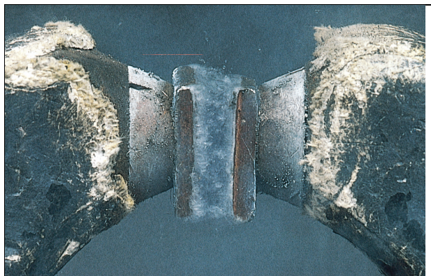
Kapalný kyslík se vznáší mezi dvěma čely magnetu, neboť je paramagnetický a je do magnetického pole vtahován.
