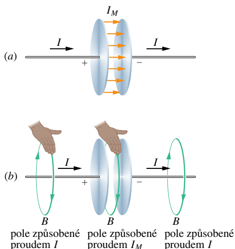
Obr. 32.17 (a) Maxwellův proud I_M mezi deskami kondenzátoru nabíjeného proudem I . (b) Pravidlo pravé ruky pro určení směru magnetického pole okolo vodiče s kondukčním (vodičným) proudem (vlevo) dává stejný směr i pro magnetické pole Maxwellova proudu (uprostřed).
