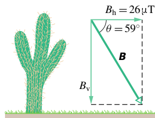
Obr. 32.6 Příklad 32.1. Zemské magnetické pole a jeho složky v Tucsonu v Arizoně v r. 1964.
