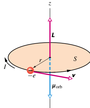
Obr. 32.8 Elektron rovnoměrně obíhá po kruhové dráze o poloměru r , která obepíná plochu S . Elektron má orbitální moment hybnosti \mathbf{L} a s ním spojený orbitální magnetický dipólový moment \boldsymbol{\mu}_{\text{orb}} . Pohyb elektronu vytváří elektrický proud I tekoucí ve směru otáčení hodinových ručiček (elektron má záporný náboj).
