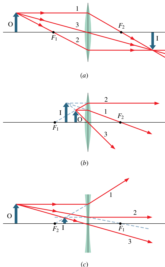
Obr. 35.15 Pomocí tří speciálních paprsků určíme polohu obrazu I vytvořeného tenkou čočkou, leží-li předmět O (a) nalevo od ohniska spojně čočky ( p > f ), (b) mezi ohniskem a spojnou čočkou ( p < f ), (c) kdekoli před rozptylnou čočkou.
