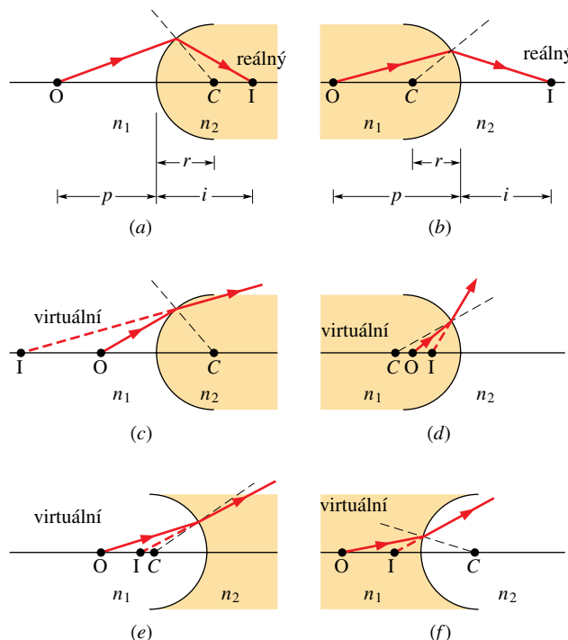
Obr. 35.11 Šest možných způsobů, při nichž vznikne obraz lomem na kulovém povrchu poloměru r se středem křivosti C. Povrch (rozhnutí) odděluje dvě prostředí s indexy lomu n_1 a n_2 . Bodový zdroj O je vždy v prostředí s n_1 nalevo od povrchu. Pro prostředí s menším indexem lomu není vystínováno (myslete si, že je to vzduch, zatímco druhé prostředí je vyplněno sklem). Reálné obrazy vznikají v případech (a) a (b), virtuální obrazy vznikají v ostatních čtyřech případech.
