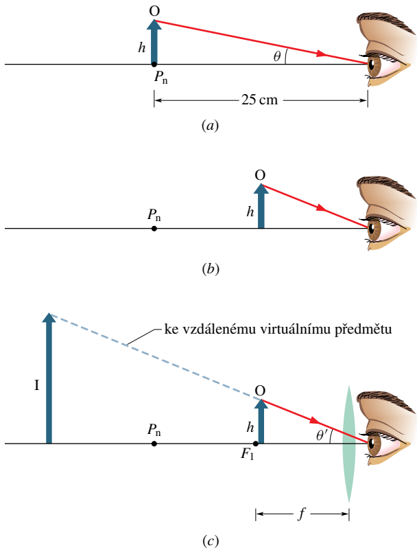
Obr. 35.17 (a) Předmět O výšky h v blízkém bodě P_n našeho oka zaujímá zorný úhel \theta . (b) Aby se zorný úhel zvětšil, posuneme předmět blíže k sobě. Pak však nedokážeme předmět zaostřit. (c) Mezi předmět a oko umístíme spojnou čočku tak, že předmět leží blízko ohniska F_1 čočky (mezi nim a čočkou). Obraz vytvořený čočkou je pak dostatečně daleko, abychom na něj mohli oko zaostřit. Zorný úhel \theta' obrazu I je nyní větší než zorný úhel předmětu O v případě (a).
