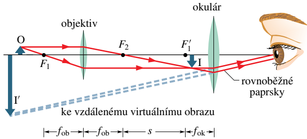
Obr. 35.18 Znárodnění mikroskopu složeného z tenkých čoček (není v měřítku). Objektív vytváří reálný obraz I předmětu O blízko ohniska F'_1 okuláru. Obraz I se pak stane předmětem pro okulár, který vytváří konečný virtuální obraz I' ; ten je prohlížen pozorovatelem. Ohnisková vzdálenost objektivu je f_{ob} , ohnisková vzdálenost okuláru je f_{ok} , délka optického intervalu (tubusu) je s .
