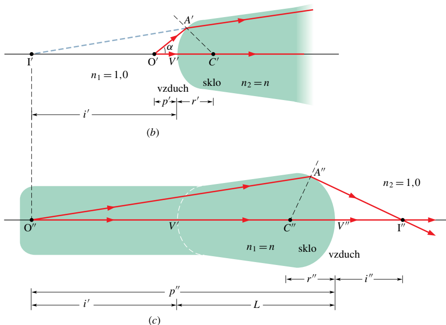
Obr. 35.22 (a) Dva paprsky vycházející z bodového předmětu O' se po lomu na dvou kulových površích „čočky“ protínají v bodě I'' — reálném bodovém obraze. Předmět leží před vypuklým povrchem na levé straně a vydutým povrchem na pravé straně čočky. Paprsek jdoucí body A' a A'' prochází ve skutečnosti čočkou po dráze blízké ose. Lomy (b) na levém povrchu a (c) na pravém povrchu jsou nakresleny odděleně.
