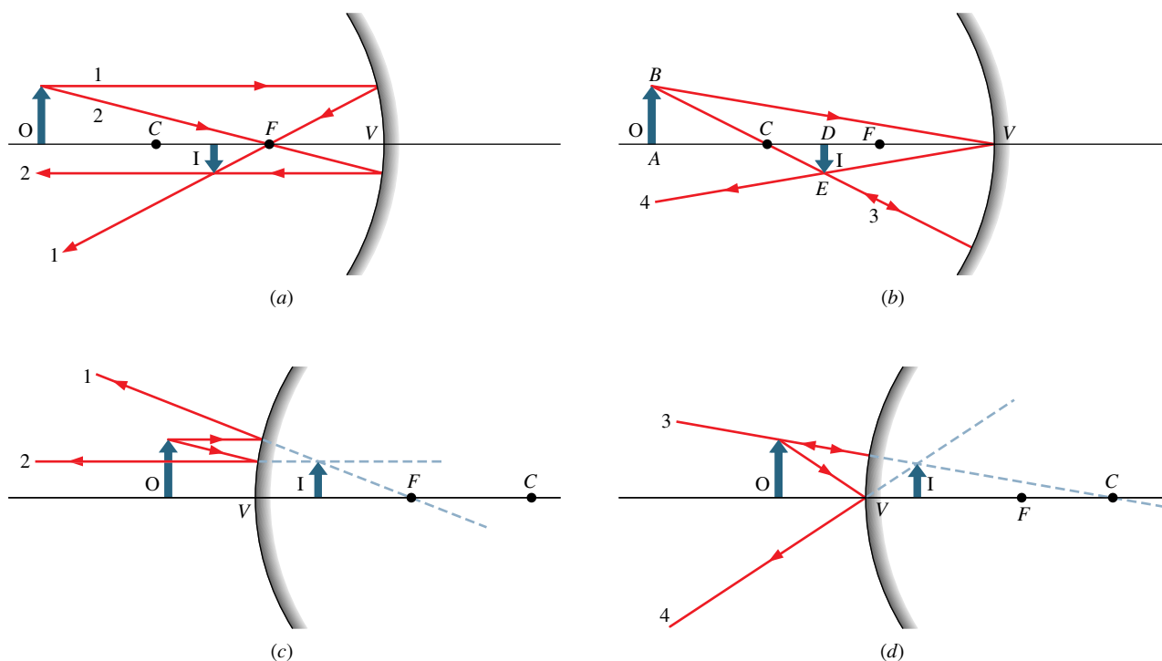
Obr. 35.10 (a, b) Čtyři paprsky, jejichž narýsováním můžeme nalézt obraz libovolného předmětu vytvořený vydutým zrcadlem. Pro polohu předmětu na obrázku vznikne reálný a převrácený obraz menší než předmět. (c, d) Čtyři podobné paprsky pro případ vypuklého zrcadla. Toto zrcadlo vytvoří vždy virtuální obraz orientovaný stejně jako předmět a menší než předmět. (Paprsek 2 v obr. (c) směřoval původně do ohniska F .)
