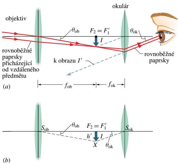
Obr. 35.19 (a) Schéma refrakčního dalekohledu složeného z tenkých čoček. Objektív vytváří reálný obraz I vzdáleného světelného zdroje (předmětu); paprsky vstupující do objektívu jsou přibližně rovnoběžné. (Předpokládáme, že jeden konec předmětu leží na centrální ose.) Ve společných ohniscích F_2 a F_1' vzniká obraz I , který je předmětem pro okulár; okulár vytváří ve velké vzdálenosti od pozorovatele konečný virtuální obraz I' . Objektív má ohniskovou vzdálenost f_{ob} , okulár má ohniskovou vzdálenost f_{ok} . (b) Obraz I má výšku h' = |F_2 X| ; paprsek S_{ob} X svírá s osou úhel \theta_{ob} , paprsek X S_{ok} svírá s osou úhel \theta_{ok} .
