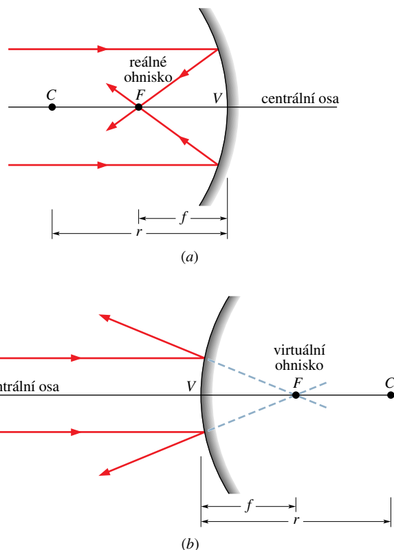
Obr. 35.8 (a) Vyduté zrcadlo soustředí dopadající rovnoběžné paprsky do reálného ohniska F , které leží na téže straně jako paprsky. (b) Vypuklé zrcadlo odráží dopadající rovnoběžné paprsky tak, jako by se rozbíhaly z virtuálního ohniska F , ležícího na opačné straně zrcadla.
