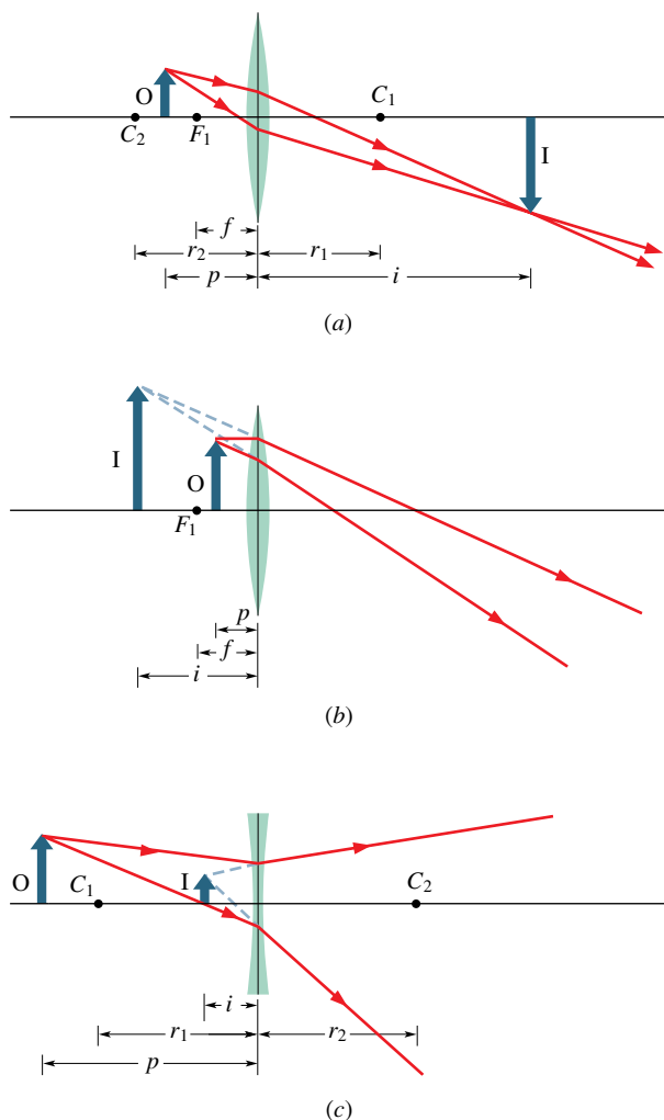
Obr. 35.14 (a) Reálný převrácený obraz I vytvoří spojná čočka tehdy, je-li předmět O umístěn před ohniskem F_1 spojně čočky (nalevo od něj). (b) Obraz I je virtuální a má stejnou orientaci jako O , je-li O mezi ohniskem a čočkou (napravo od F_1 ). (c) Rozptylná čočka vytváří virtuální obraz I stejně orientovaný jako předmět O nezávisle na tom, zda předmět leží nalevo od ohniska nebo napravo od něj.
