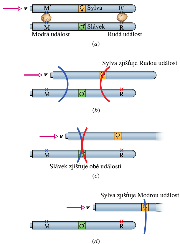
Obr. 38.4 Kosmické lodě Sylvy a Slávka a události ze Slávkovy pohledu. Sylvina loď letí napravo rychlostí \mathbf{v} . (a) Rudá událost nastává v místech R, R' a Modrá v místech M, M'. Každá z nich vysílá svou světelnou vlnu. (b) Sylva zjišťuje vlnu od Rudé události. (c) Slávek zjišťuje vlny od obou událostí současně. (d) Sylva zjišťuje vlnu od Modré události.
