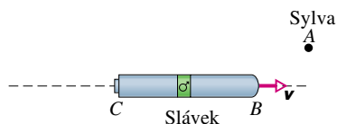
Obr. 38.8 Příklad 38.4. Sylva měří, jak dlouho trvá loď, když ji v bodě A mĕří.
