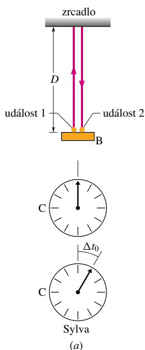
Obr. 38.5 (a) Sylva, sedící ve vlaku, měří dobu \Delta t_0 mezi událostmi 1 a 2 jedinými hodinami C ve vlaku. Údaj hodin je ukázán dvakrát: nejprve pro událost 1, pak pro 2. (b) Slávek, pozorující děj ze stanice, potřebuje dvoje synchronizované hodiny — C_1 pro událost 1 a C_2 pro událost 2. Naměří jimi dobu \Delta t .
