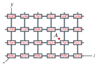
Obr. 38.3 Řez trojrozměrným polem hodin a měřicích tyčí, kterými pozorovatel může přiřadit události její prostorčasové souřadnice. Záblesk světla (bod A) má souřadnice zhruba x = 3,7 tyčí, y = 1,2 tyčí, z = 0 . Časovou souřadnici udávají ty hodiny, které jsou v daném okamžiku v těsné blízkosti události A.
