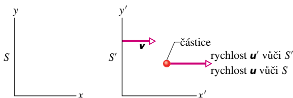
Obr. 38.12 Vztažná soustava S' se pohybuje rychlostí \mathbf{v} vůči soustavě S . Částice má rychlost \mathbf{u}' vůči soustavě S' a rychlost \mathbf{u} vůči soustavě S .
