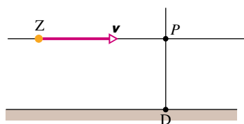
Obr. 38.13 Zdroj světla Z letí rychlostí \mathbf{v} kolem detektoru D . Podle speciální teorie relativity nastane příčný Dopplerův jev, když zdroj prochází bodem P . Jeho rychlost je tam kolmá na spojnici ZD . Podle klasické teorie by Dopplerův jev v takovém případě nastat neměl.
